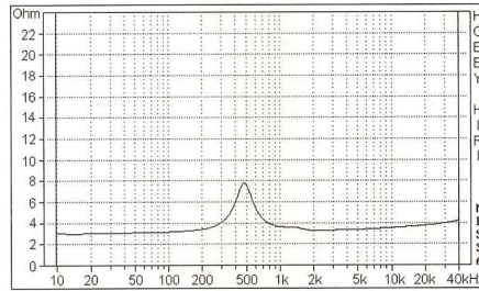
Impedanz-Frequenzgang Sehr niedrige Schwingpuleninduktivität, Anflug eines Ventilationsproblems bei 1,5 kHz.
