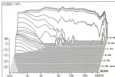
Wasserfallspektrum Halbraum axial Allerbestes transientes Verhalten.
